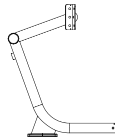
5. PLC Pivot Frame QTY 1
