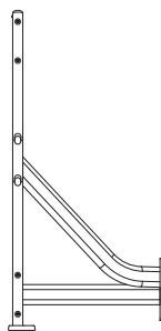
3. PTD ASSY, ODB LEFT UPRIGHT QTY 1
