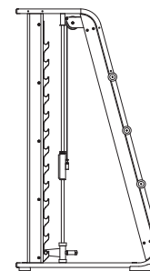
2. Assy, Sm Left Side QTY 1
