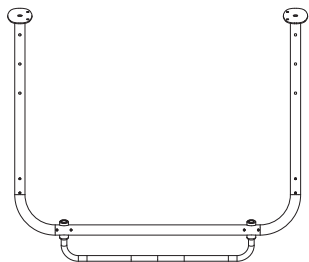
13. Top Frame QTY 1
