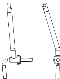
9. Left Handle Arm QTY 1
